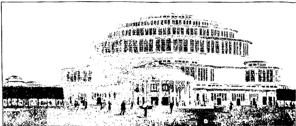
NEUE FESTHALLE, genannt „JAHRHUNDERTHALLE“, aus Beton und Eisenbeton: lichte Weite der Kuppel 65 m, größte Kuppelspannweite der Welt. Höhe des Kuppelraumes 40 m, lichte Weite des Halleninneren 95 m. Fassungsvermögen 9000 Personen
