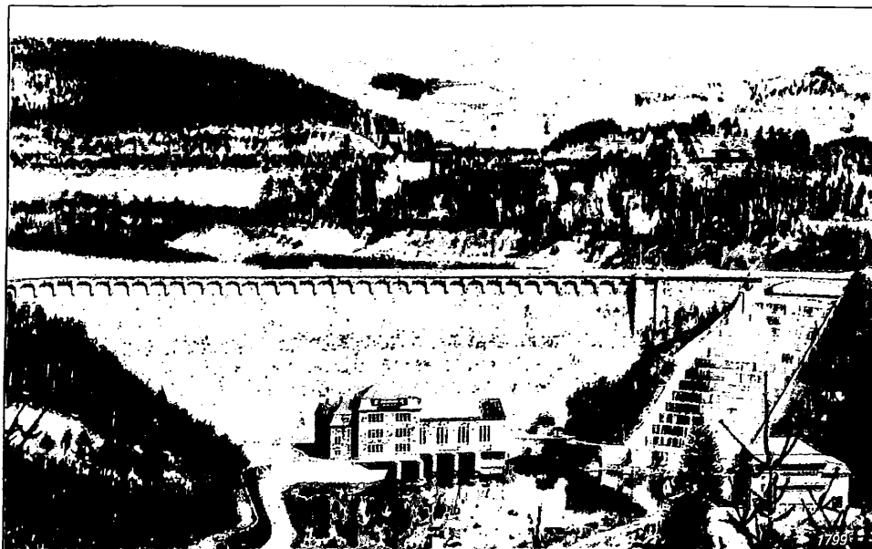
Die Talsperre bei Mauer a. Bober. Die Mauerlänge betrug unten 140 und oben 280 Meter, die Mauerbreite unten 51 oben 7,2 Meter, die Mauerhöhe 60 Meter und das Stau-becken faßt 50 Millionen cbm Wasser
